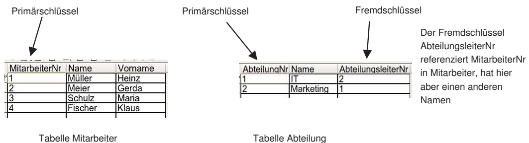
Abbildung 4.12: Auflösung der 1:1-Beziehung Mitarbeiter-Abteilung
