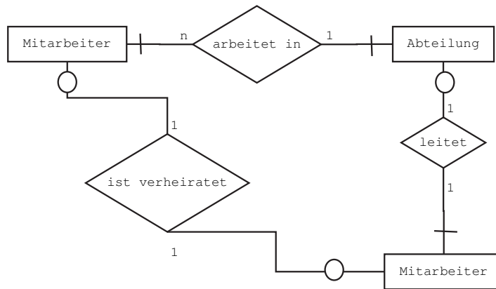
Abbildung 3.16: ERM: Nicht Redundante Beziehung
