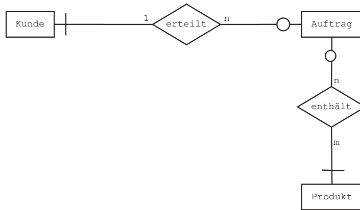
Abbildung 3.18: ERM Beispiel 3.1 Gesamtdarstellung
