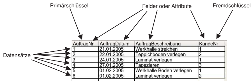
Abbildung 2.3: Die Tabelle Auftrag
